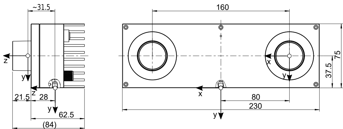
Abb. 3.8: Ungefähre Position des Sensor-/Kamerakoordinatensystems (in der linken Kameralinse) und des Montagepunkt-Koordinatensystems (am Stativgewinde) für den rc_visard NG 160
