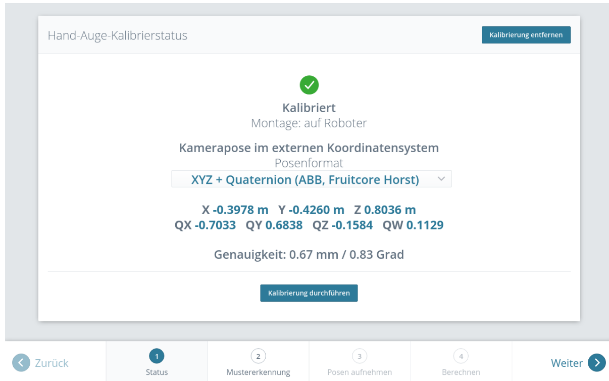
Abb. 6.21: Aktueller Status der Hand-Auge-Kalibrierung falls eine Hand-Auge-Kalibrierung gespeichert ist
