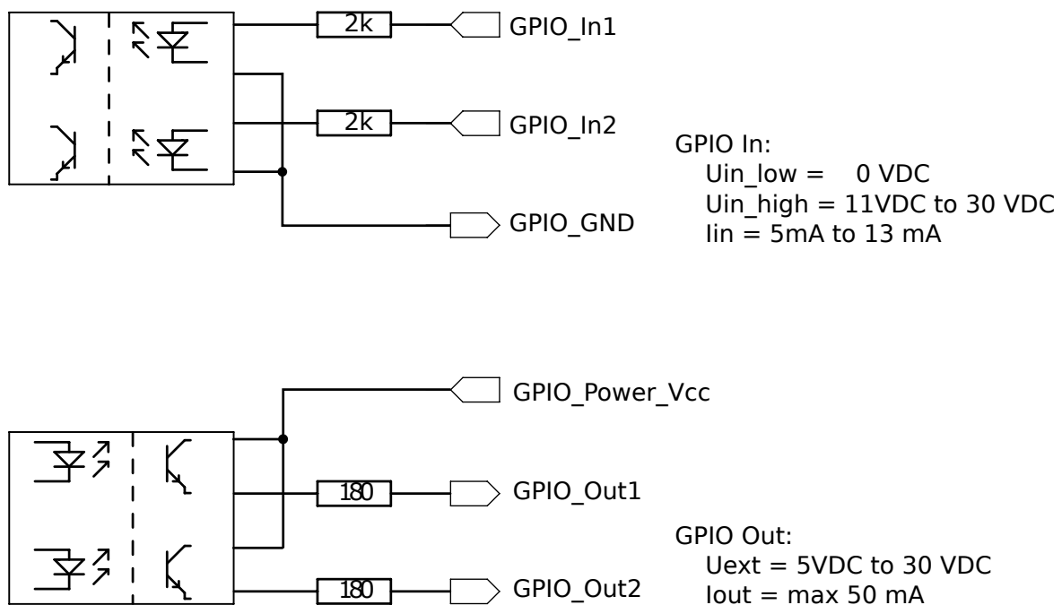
Abb. 3.6: GPIO-Schalterschema und zugehörige Spezifikationen: Keine Signale über 30 V anschließen!
