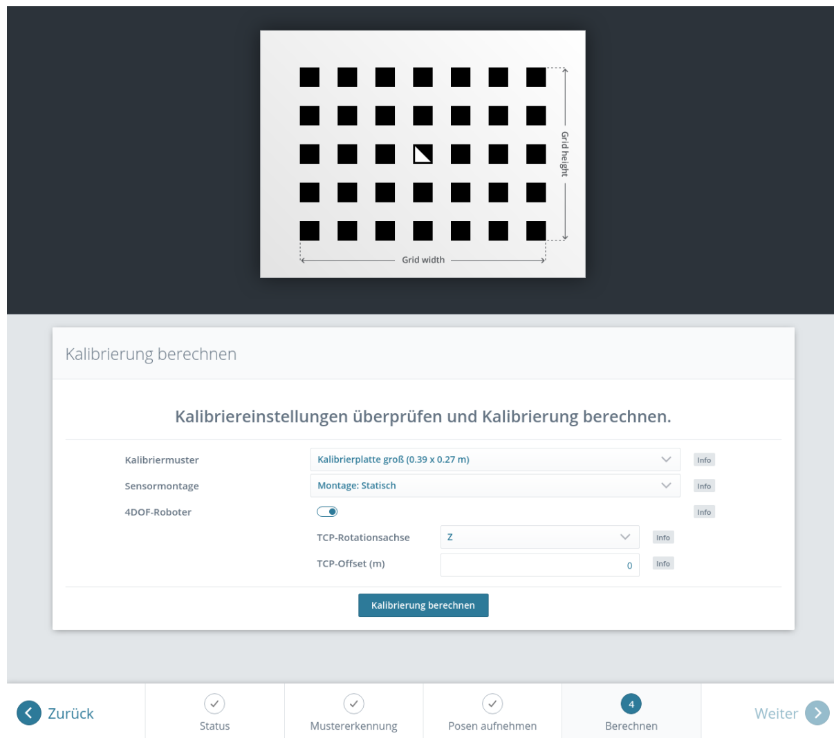
Abb. 6.25: Setzen der Parameter und Berechnen der Hand-Auge-Kalibrierung in der Web GUI des rc_visard NG
