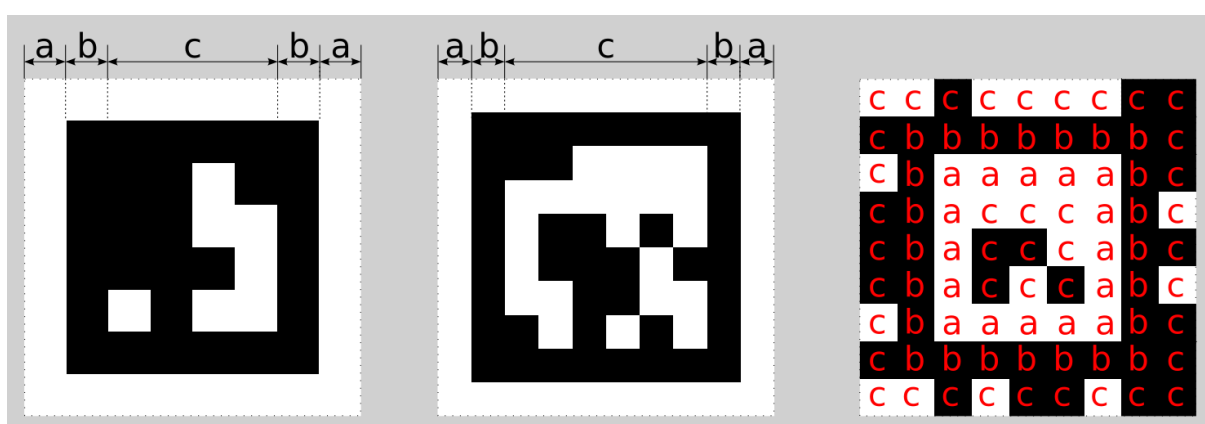
Abb. 6.8: Ein 16h5 Tag (links), ein 36h11 Tag (Mitte) und ein 41h12 Tag (rechts). AprilTags bestehen aus einem obligatorischen weißen (a) und schwarzen (b) Rahmen und einer variablen Menge an Datenmodulen (c).
