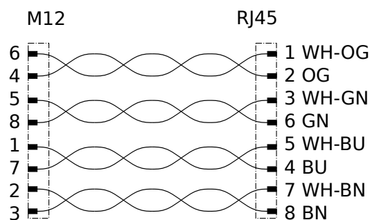
Abb. 3.5: Steckerbelegung für die M12/Ethernet-Verkabelung
