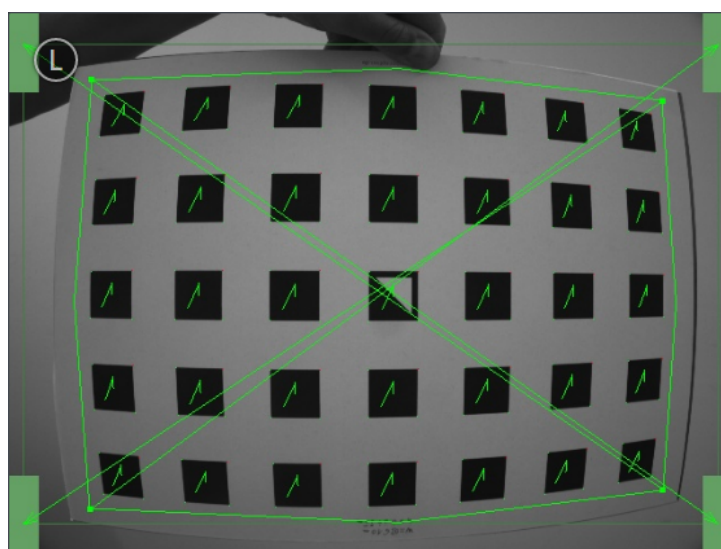
Abb. 6.32: Wird das Kalibrieremuster falsch herum gehalten, kreuzen sich die grünen Linien.
