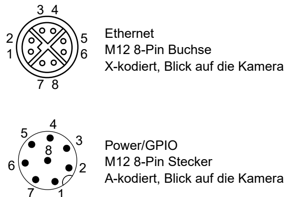
Abb. 3.4: Steckerbelegung für den Strom- und Ethernetanschluss
