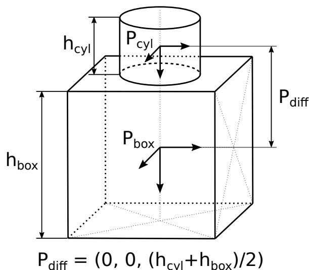
Abb. 6.42: Bezugssysteme für das Erstellen von Greifern über die REST-API und die Web GUI
