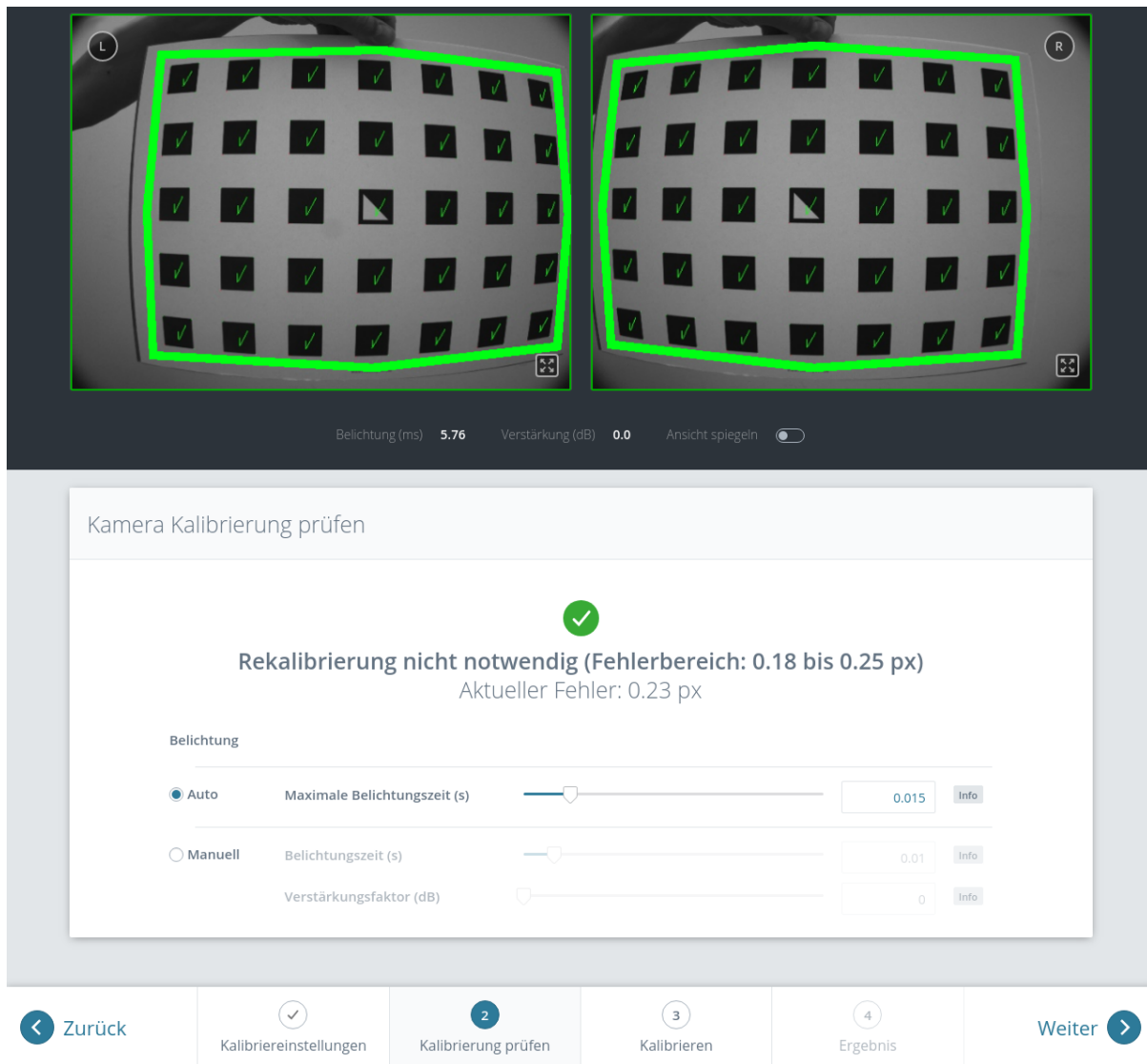
Abb. 6.28: Überprüfung der Kalibrierung
