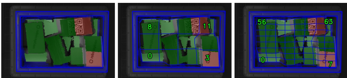
Abb. 6.6: Visualisierungen des Behälterfüllstands: Gesamtfüllstand ohne Raster (links), 4x3 Raster (Mitte), 8x8 Raster (rechts). Der Inhalt wird mit einem Farbverlauf von weiß (auf dem Boden) nach dunkelgrün dargestellt. Die überfüllten Bereiche sind rot dargestellt. Die Nummern stellen die Zell-IDs dar.
